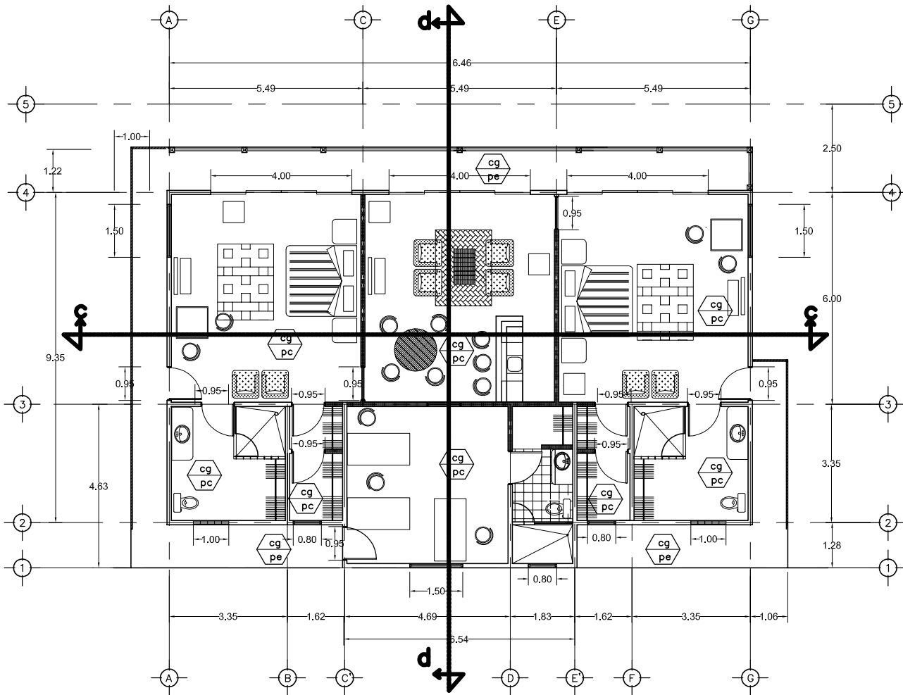
Planta Arquitectonica
